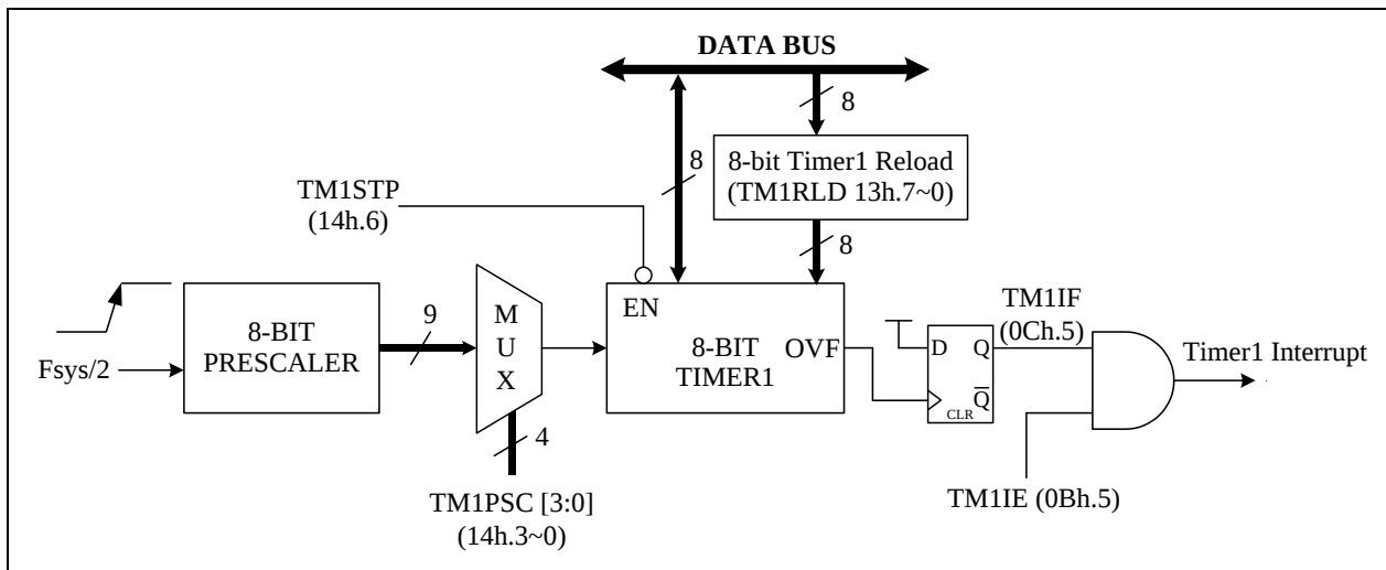
Timer1 框图
