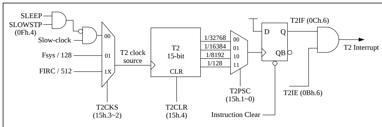
T2 框图
