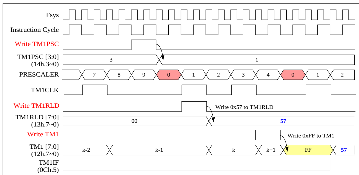
Timer1 时序图
