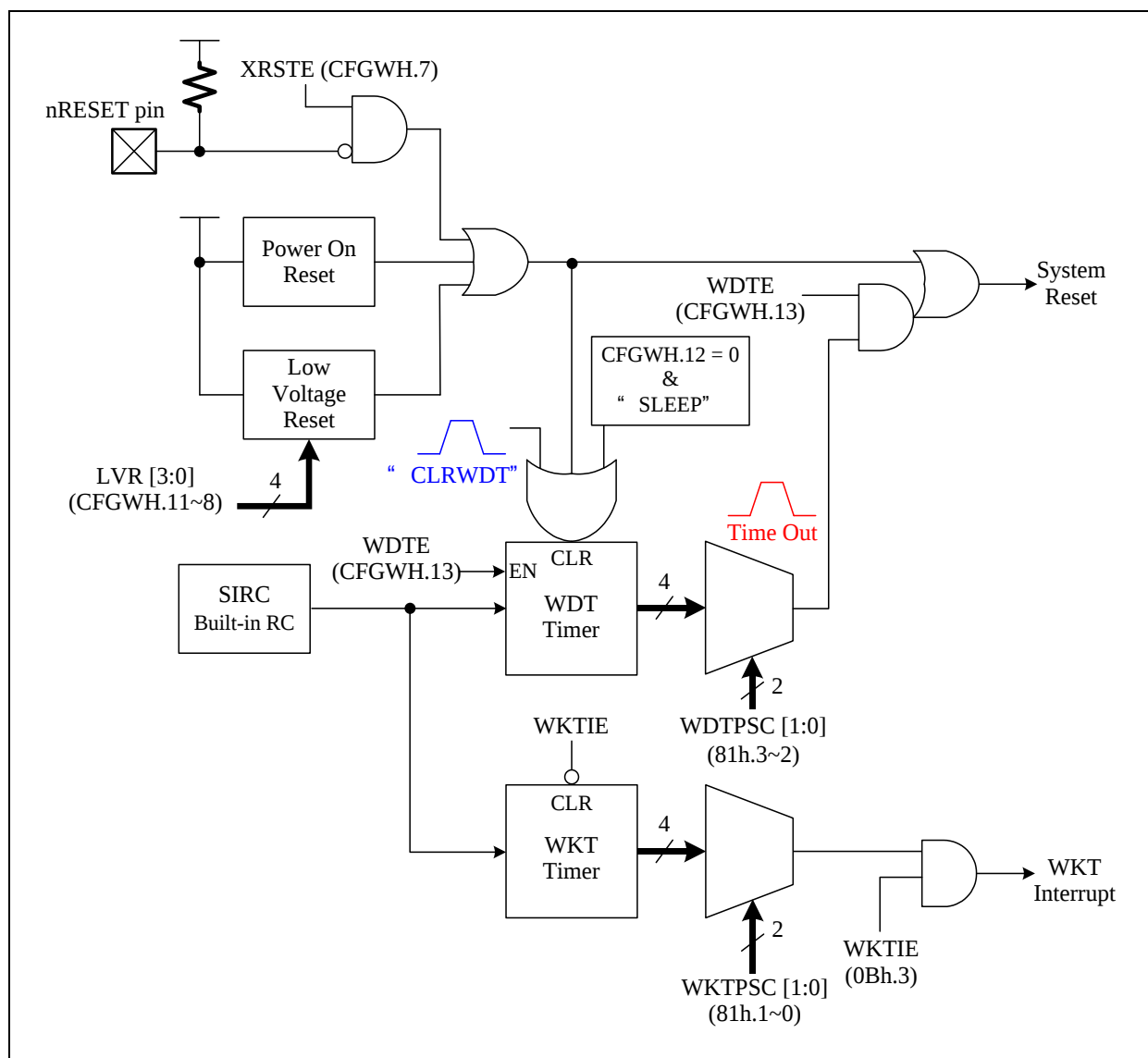
WDT/WKT 框图
