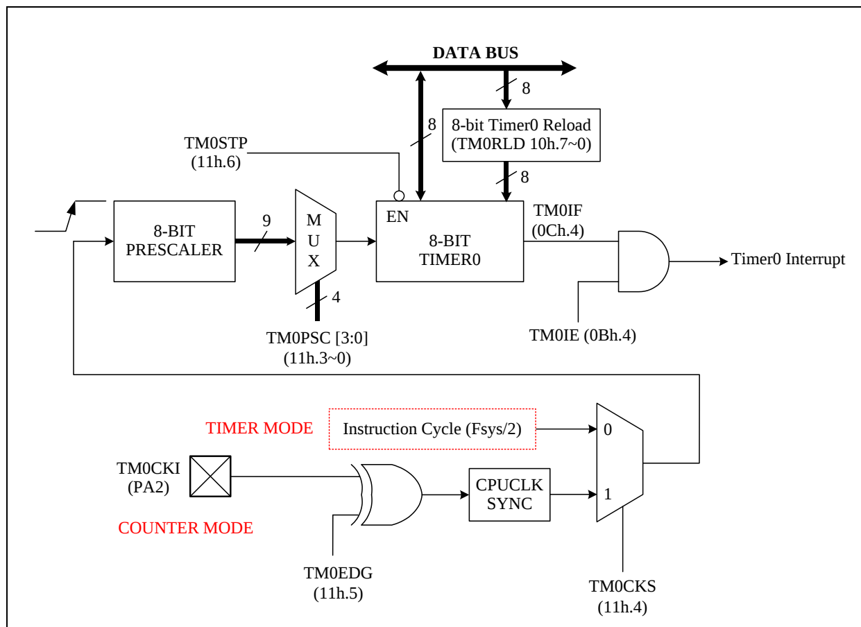
Timer0 框图
