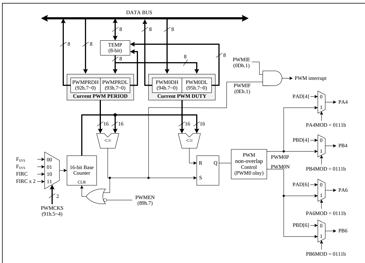
PWM0 框图
