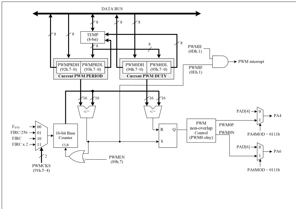
PWM0 框图
