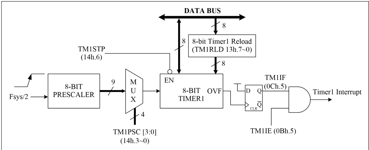
Timer1 框图
