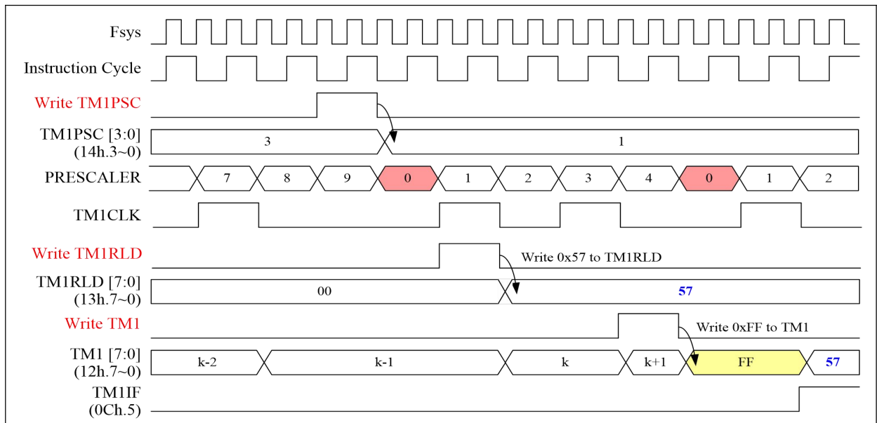
Timer1 时序图
