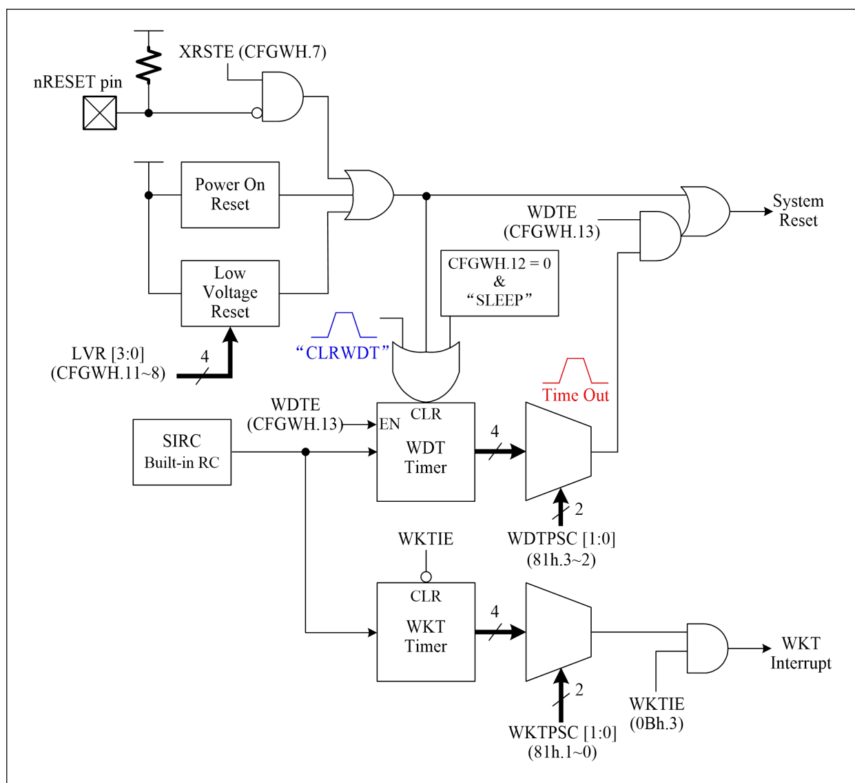
WDT/WKT 框图
