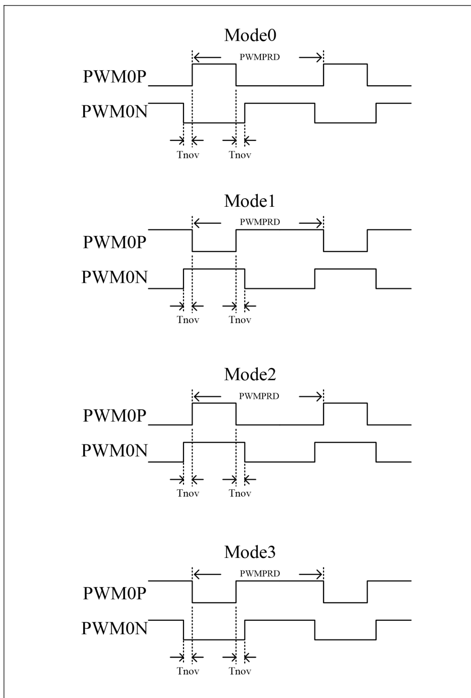
PWM0 时序图
