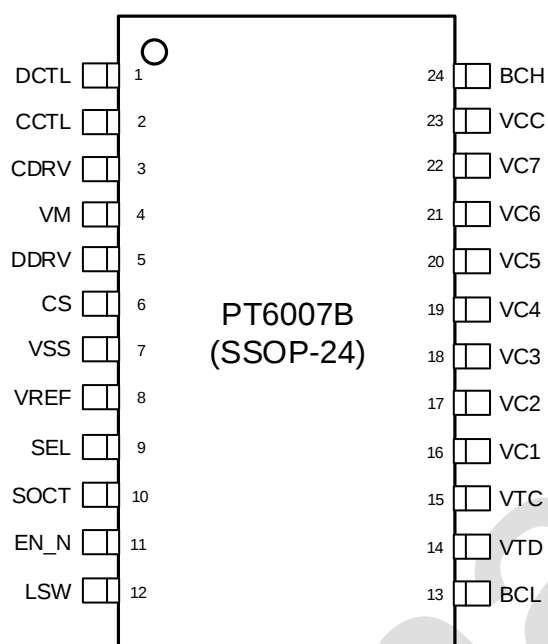
图 3. 管脚定义图
