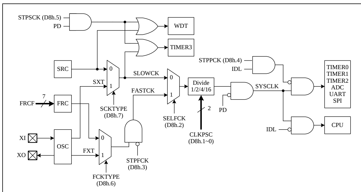
时钟结构
