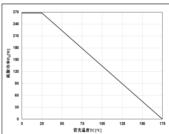
图 17 耗散功率-壳温 T_c 特性 ( T_J \leq 175^\circ C )
