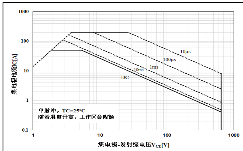
图 19 正向安全工作区
