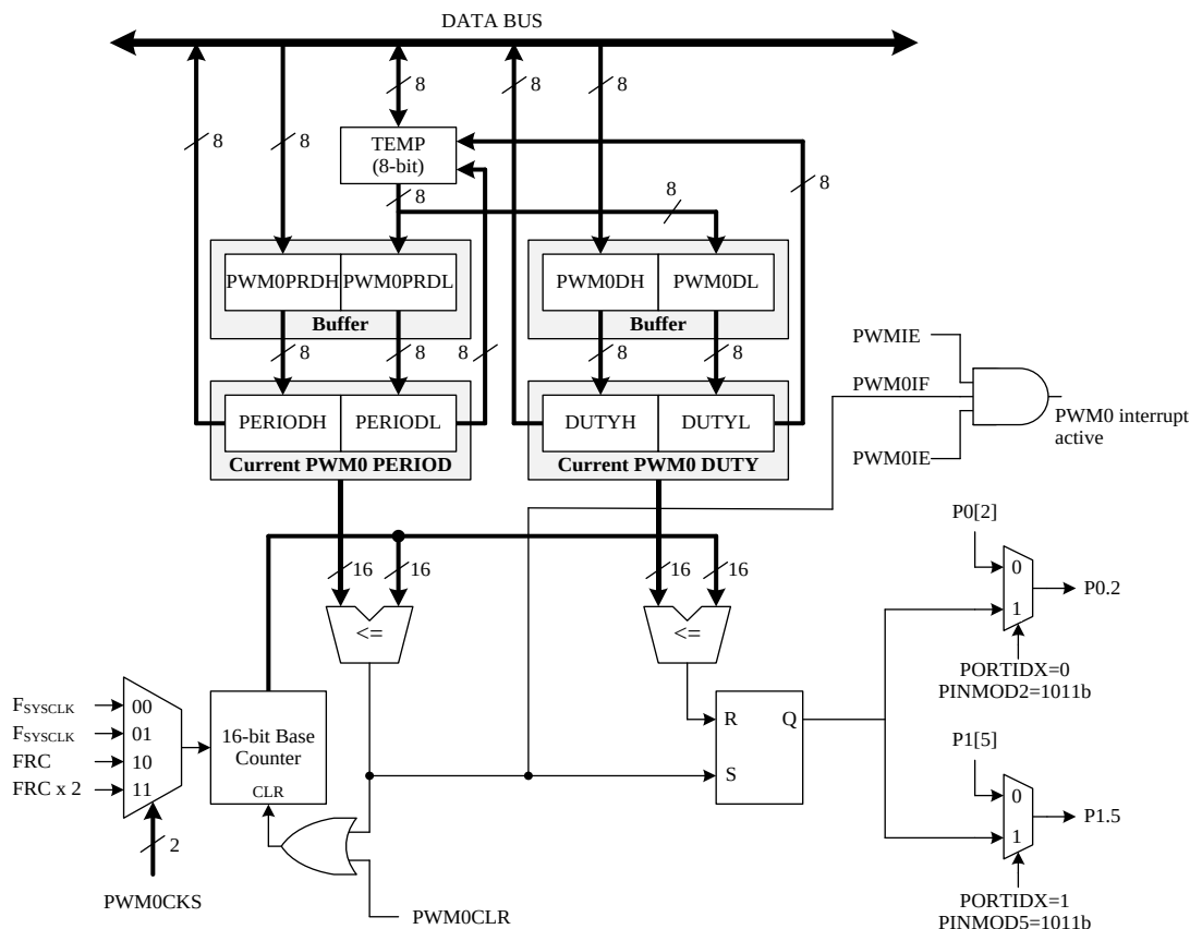
PWM0 结构
